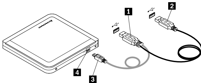
Abbildung 2. Laufwerk anschließen
