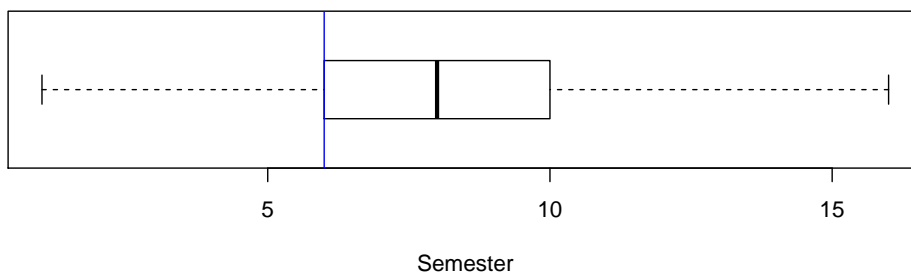
Abbildung 3: Studiendauer
