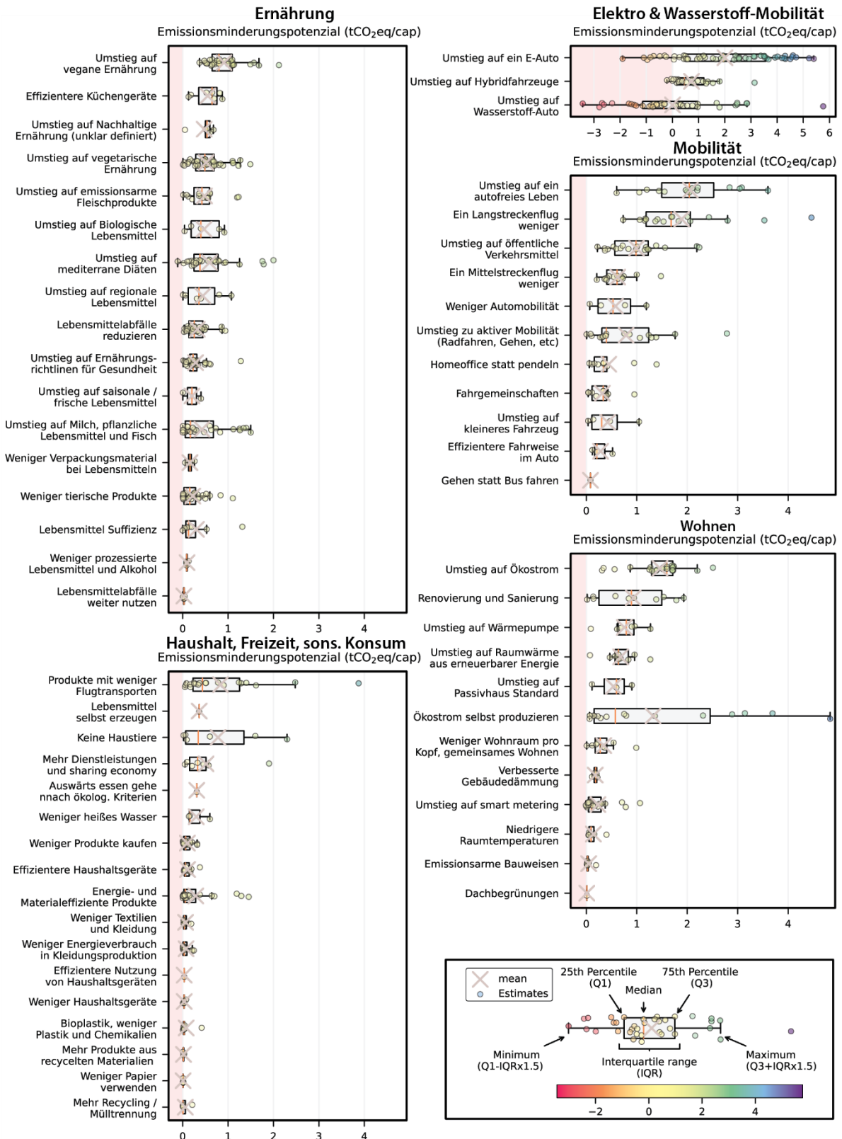
Abbildung 3.1: Die internationalen Emissionsvermeidungs- und -verringierungspotenziale von 60 Konsumoptionen. Eigene Darstellung adaptiert nach Ivanova et al (Ivanova et al., 2020).
