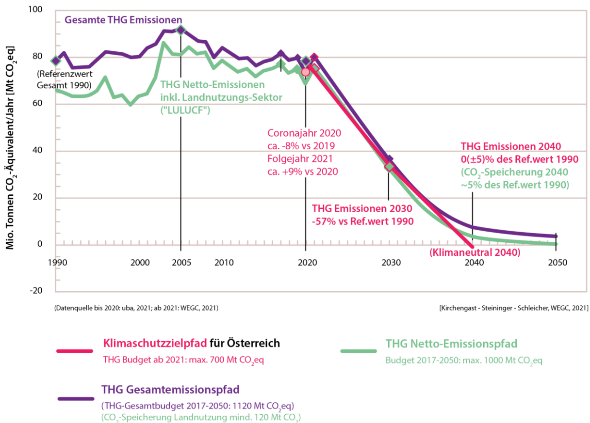
Abbildung 12.2: Emissionsreduktionspfad zur Erreichung des Pariser Klimaziels in Österreich 11
